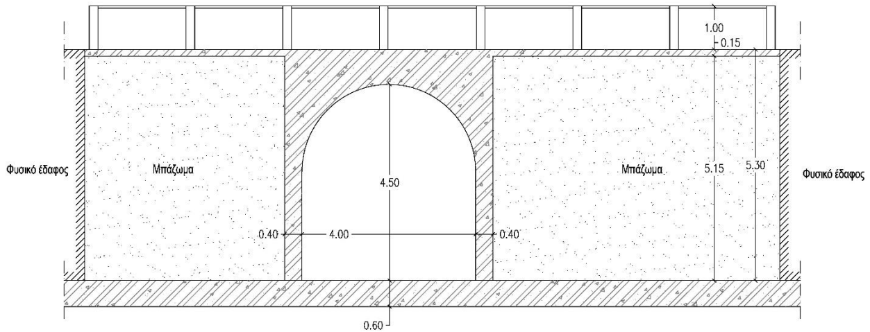
Τομή Α-Α
