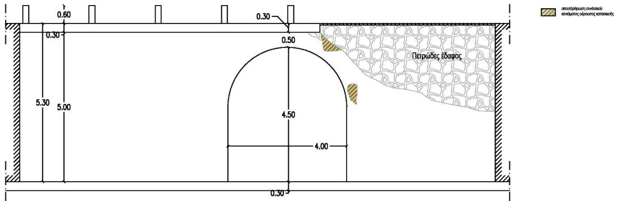
Νοτιανατολική όψη
