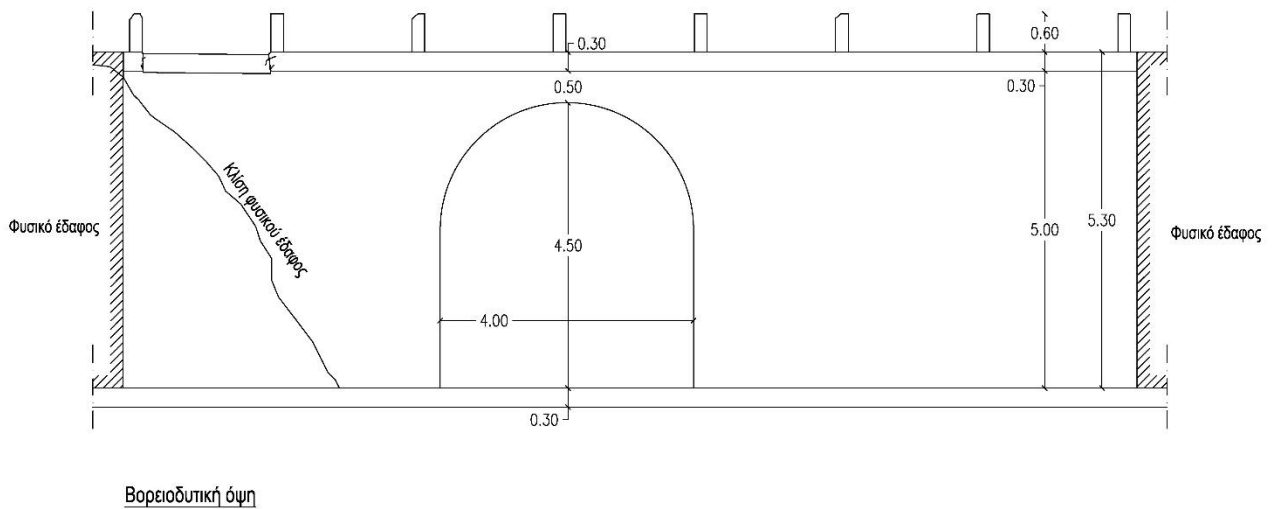
Εικόνα 3: σκαρίφημα Βορειοδυτικής όψης γεφυριού
