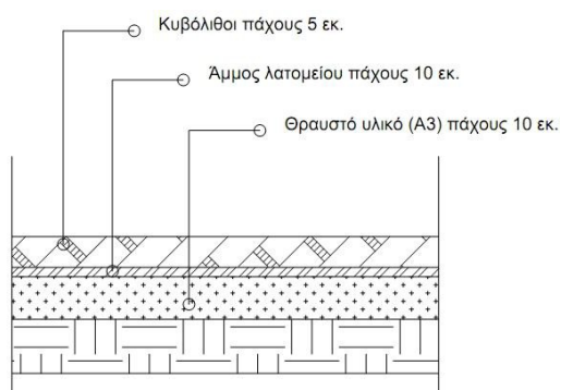
Εικόνα: Τομή ενδεικτικής εφαρμογής κυβόλιθου.
