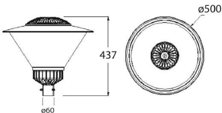
Εικόνα: Ενδεικτική διάταξη φωτιστικού
